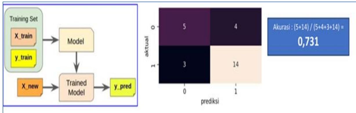
Gambar2. Skema pengukuran akurasi prediksi machine learning
